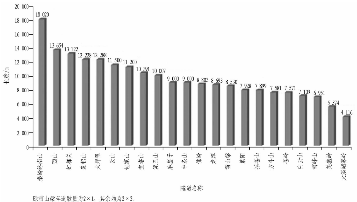
(a) 山岭公路隧道
